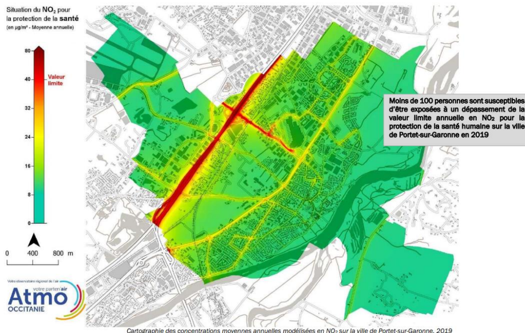
Cartographie des concentrations moyennes annuelles modélisées en NO 2 sur la ville de Portet-sur-Garonne, 2019
